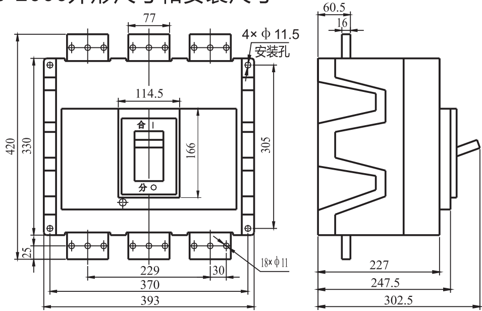
图2 DZ20J-2000板前接线外形尺寸和安装尺寸
