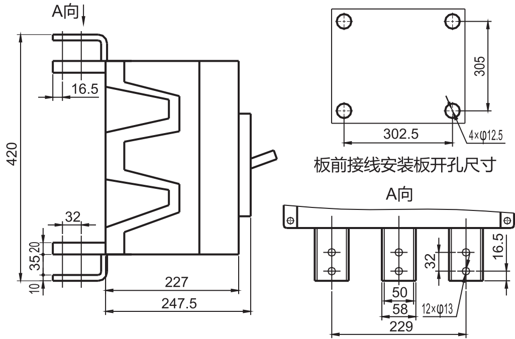
图2 板后接线外形尺寸和安装尺寸
