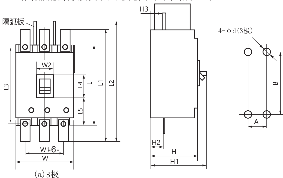
图1 板前接线外形及安装尺寸
