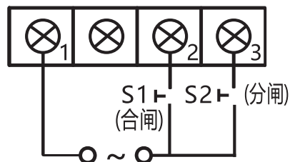
图5a CD型电动操作机构接线图
