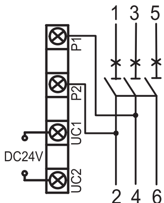
图1 DC24V接线图
