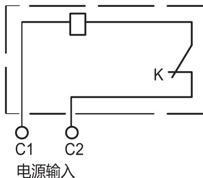
图2 AC50Hz、230V、400V接线图
