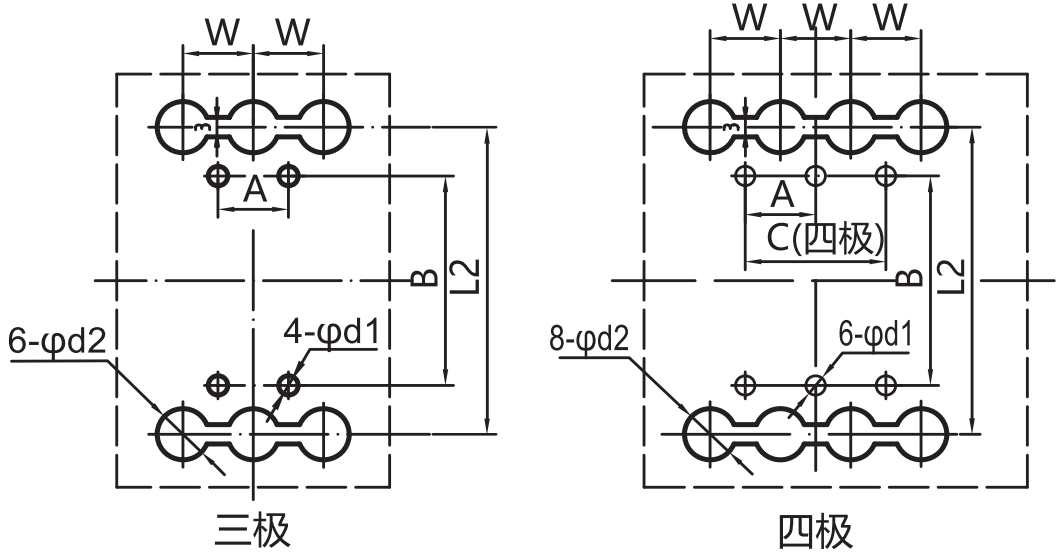
图9 RDM1系列板后接线安装板开孔尺寸
