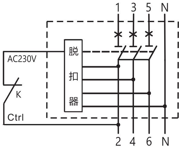
图4 费控电能表专用断路器接线图
