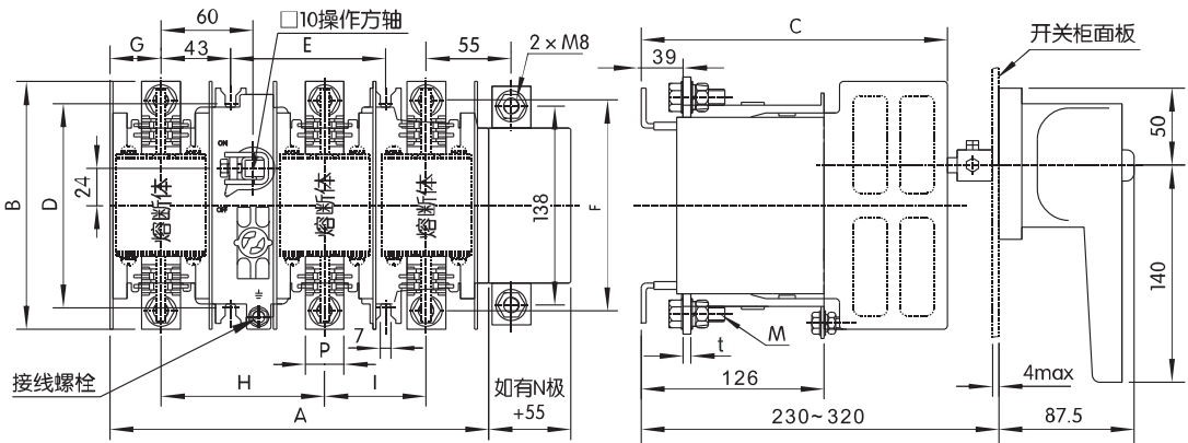
HH15(QSA)-250S、400S 外形及安装尺寸
