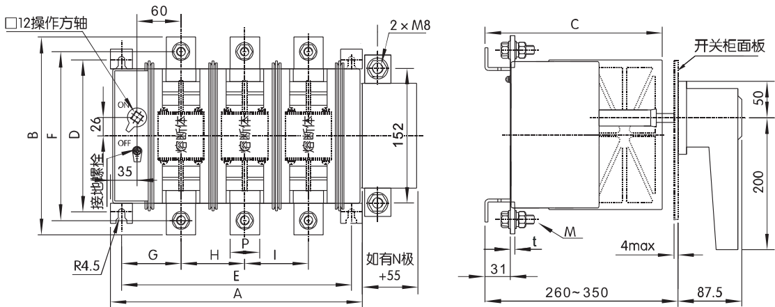
HH15(QSA)-630S、800S 外形及安装尺寸
