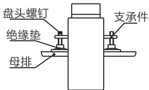
图6 母线固定
