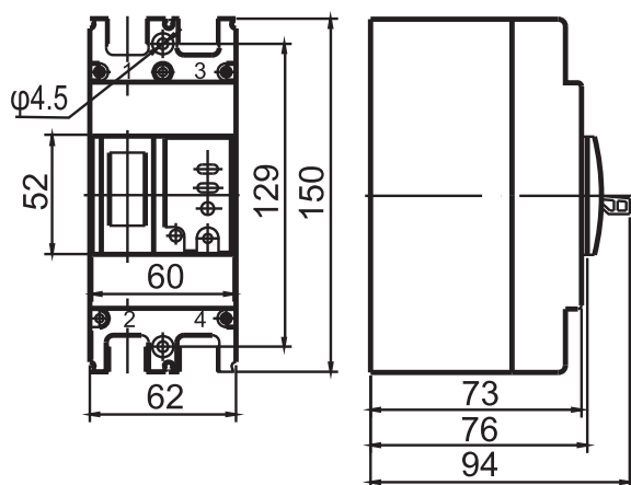
图4a RDM3L-125/2300
