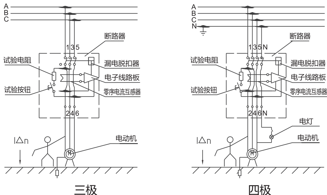
图1 工作原理
