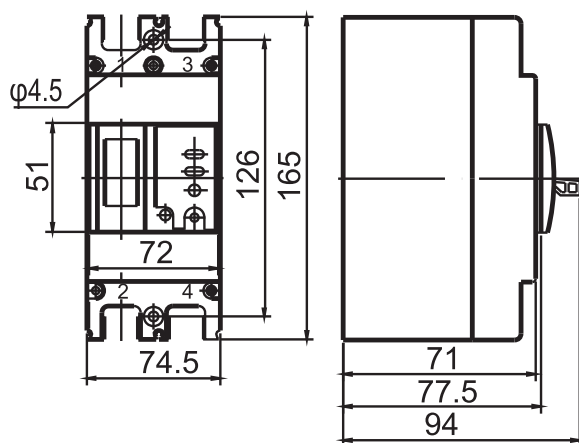
图4b RDM3L-250/2300
