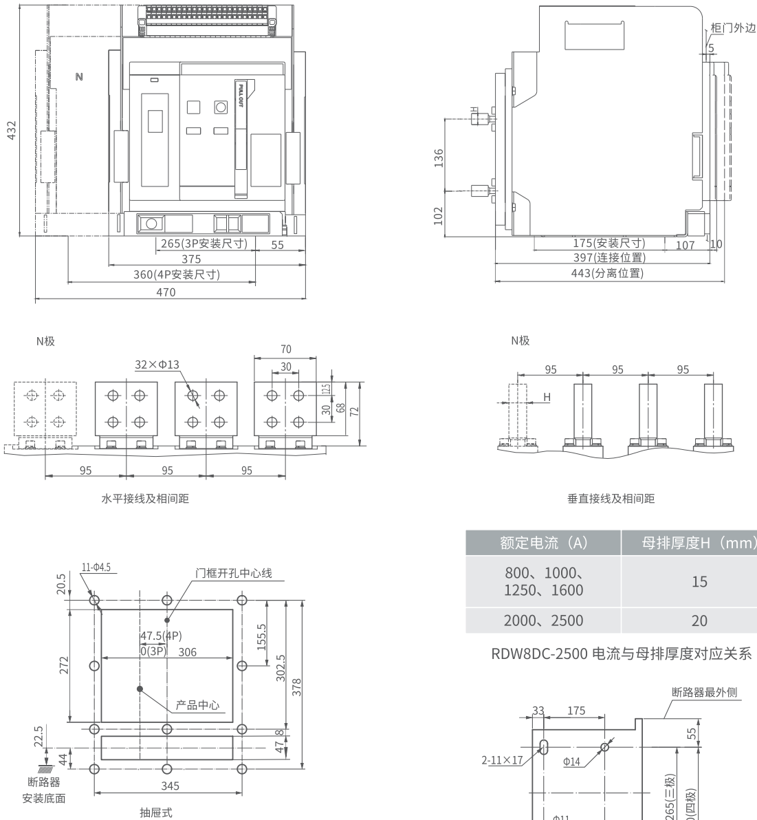
RDW8DC-2500抽屉式断路器面板开孔尺寸
