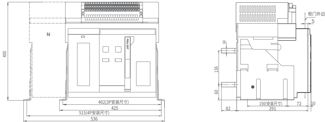
RDW8DC-4000智能型万能式断路器（固定式）
