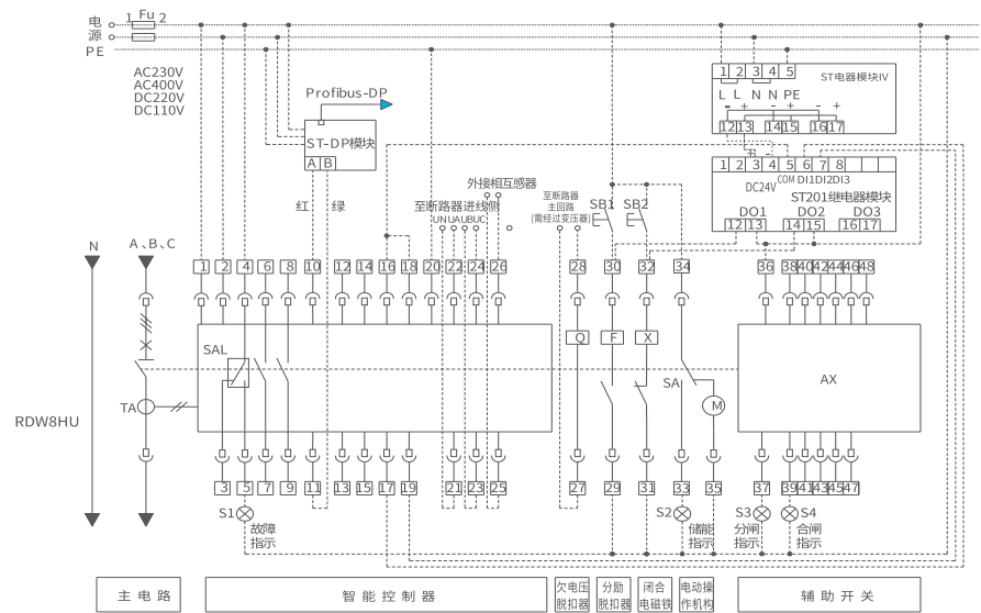
RDW8HU-2500/4000/6300带重合闸功能断路器控制回路接线图
