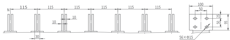
4P垂直接线及相间距
