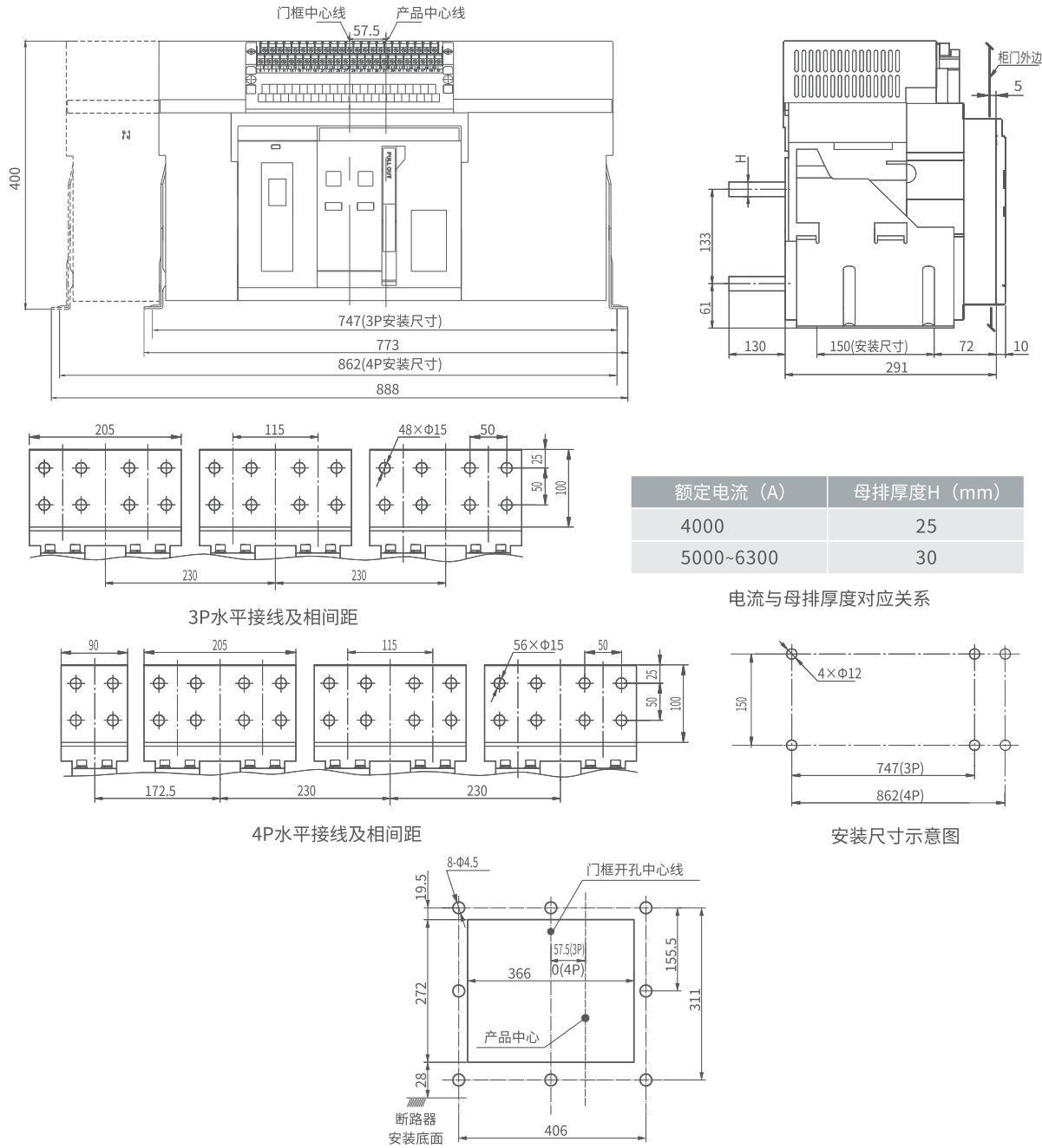
RDW8HU-6300固定式断路器面板开孔尺寸
