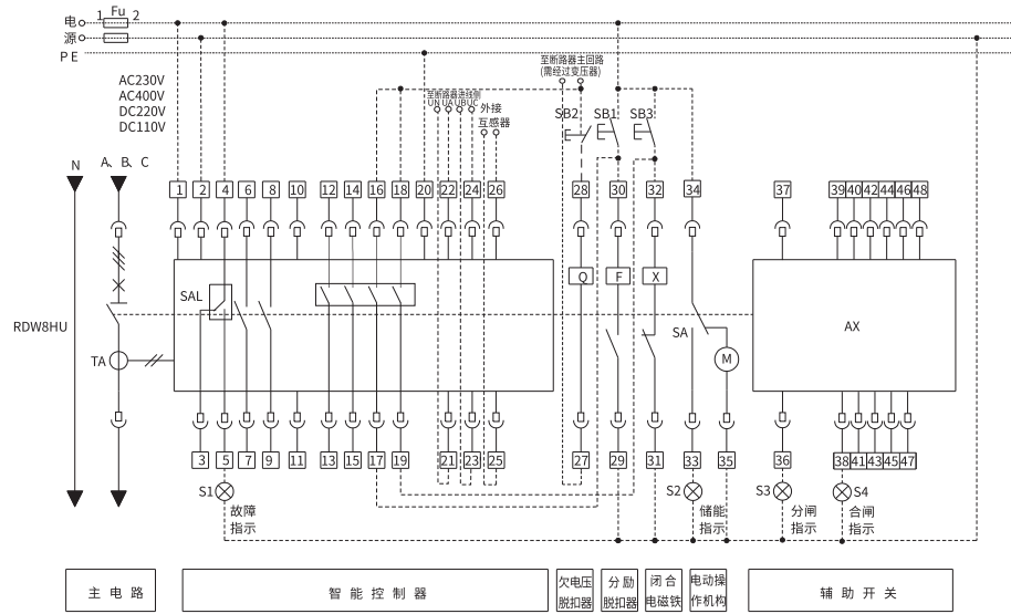
RDW8HU-2500/4000/6300带重合闸功能断路器控制回路接线图
