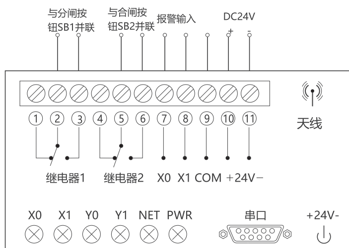
远程控制器接线图
