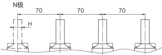
垂直接线及相间距
