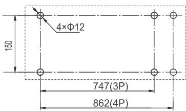
安装尺寸示意图
