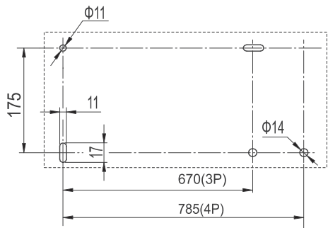
安装尺寸示意图
