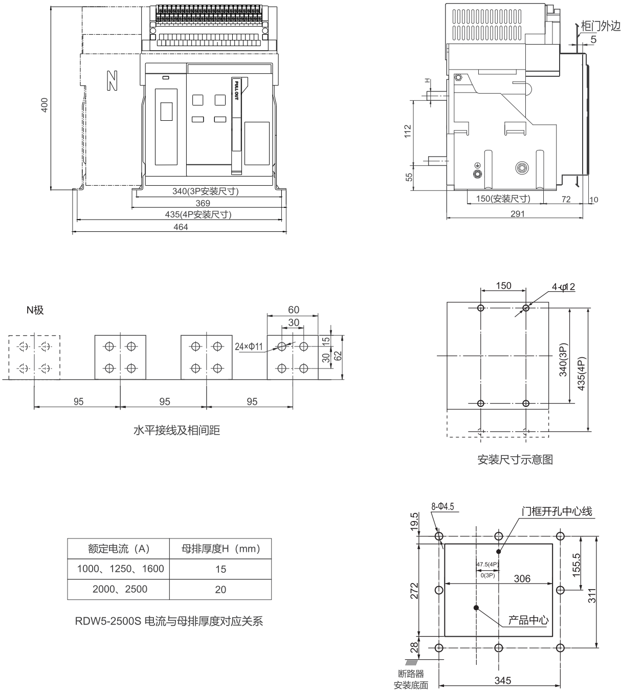
RDW5-2500S固定式断路器面板开孔尺寸
