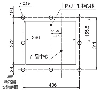
RDW5-6300H固定式断路器面板开孔尺寸
