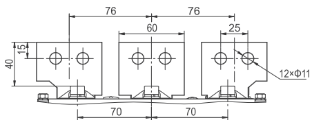
3P水平接线及相间距
