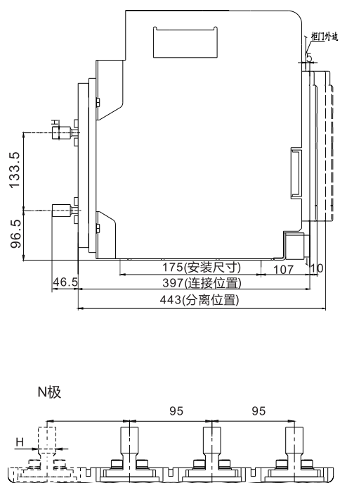
垂直接线及相间距
