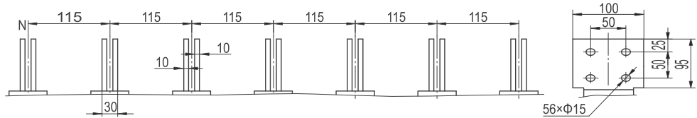
4P垂直接线及相间距
