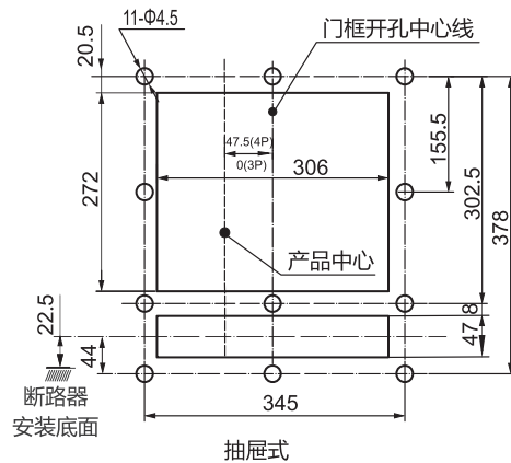
RDW5-2000S抽屉式断路器面板开孔尺寸
