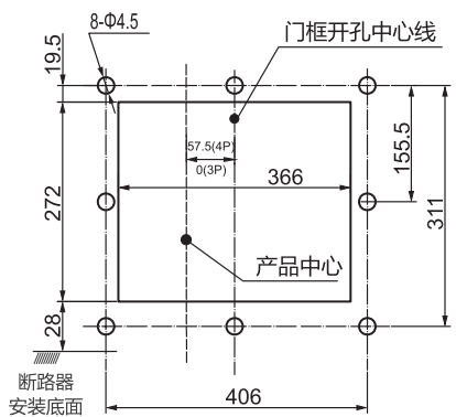
RDW5-3200S固定式断路器面板开孔尺寸
