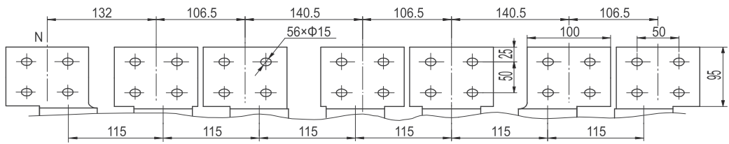
4P水平接线及相间距
