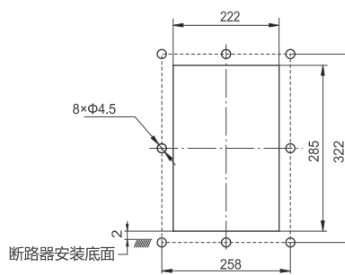
RDW5-1600H固定式断路器面板开孔尺寸
