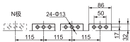
水平接线
