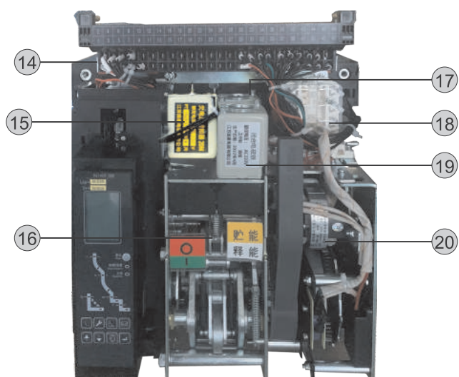
断路器本体
