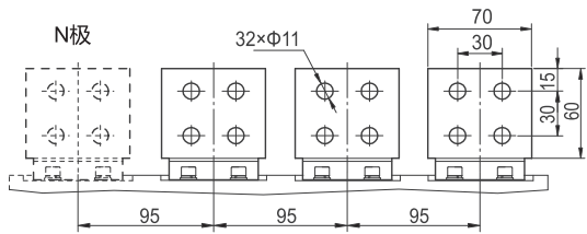
水平接线及相间距
