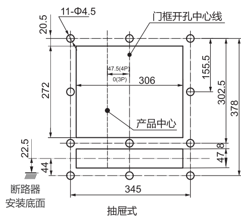
RDW5-2000H抽屉式断路器面板开孔尺寸
