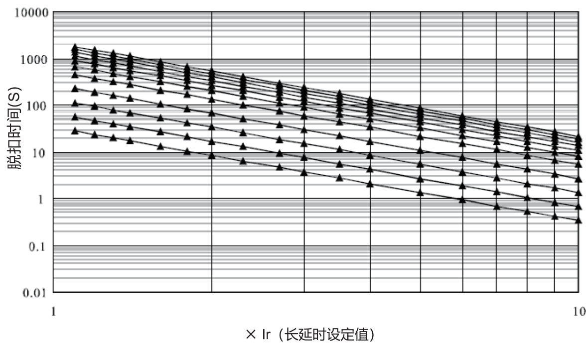
I^2T 曲线图
