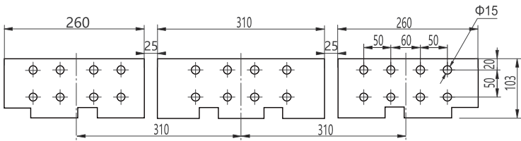
三极极水平接线及相间距
