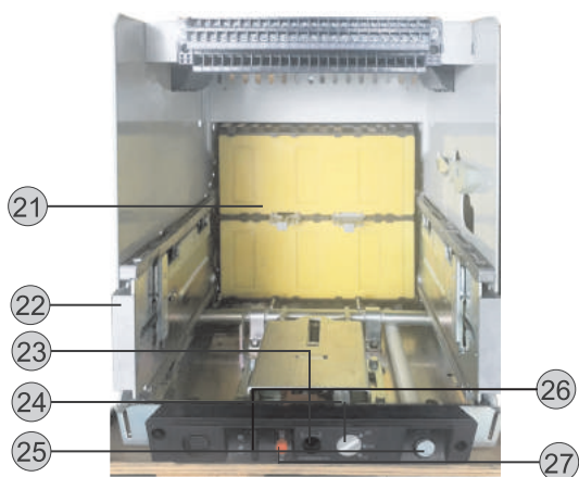
抽屉座
