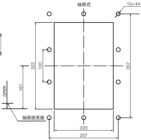
RDW5-1600H抽屉式断路器面板开孔尺寸
