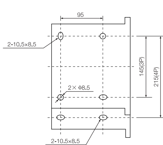
安装尺寸示意图
