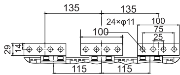
2900-3200 (3P) 水平接线
