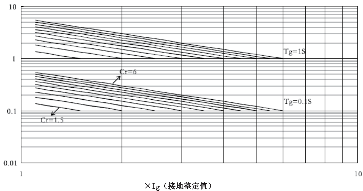
接地保护
