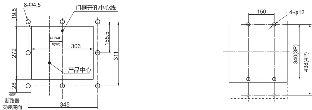
RDW5-2000H 电流与母排厚度对应关系
