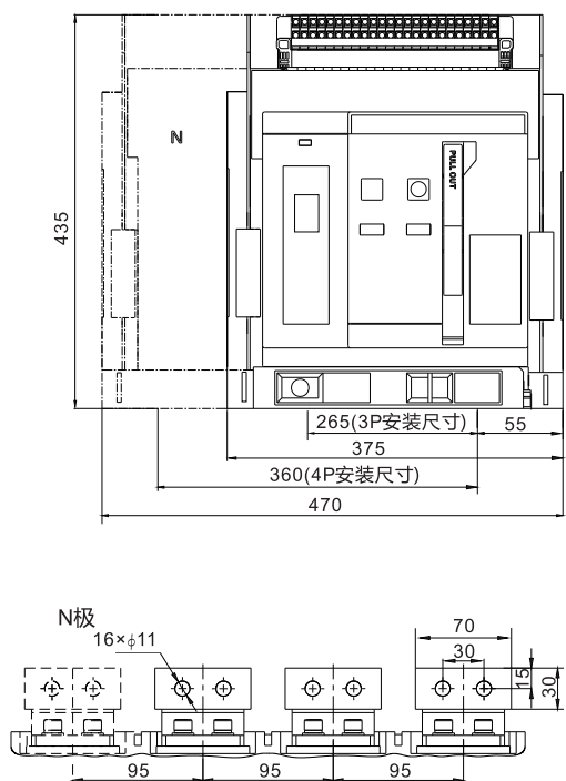
水平接线及相间距
