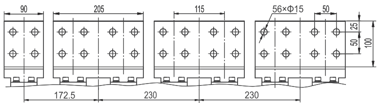
4P水平接线及相间距
