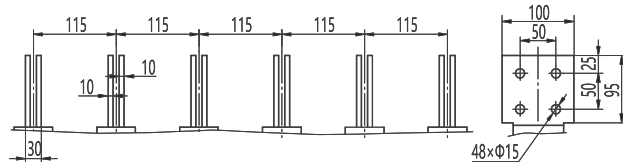
3P垂直接线及相间距
