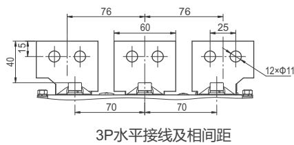
RDW5-1600H安装尺寸
