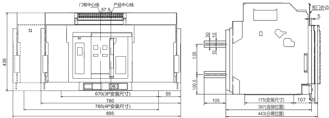
RDW5-6300H安装尺寸及面板开孔尺寸
