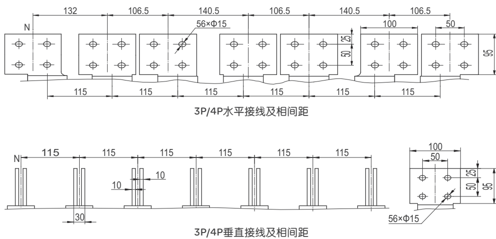
RDW5-6300H接线尺寸
