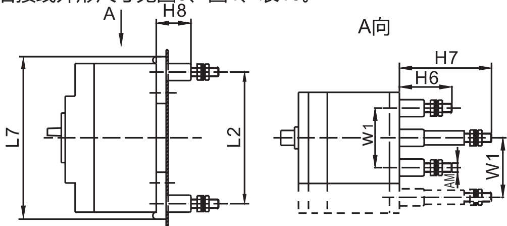
图3 RDM7E-100、125、250固定式板后接线
