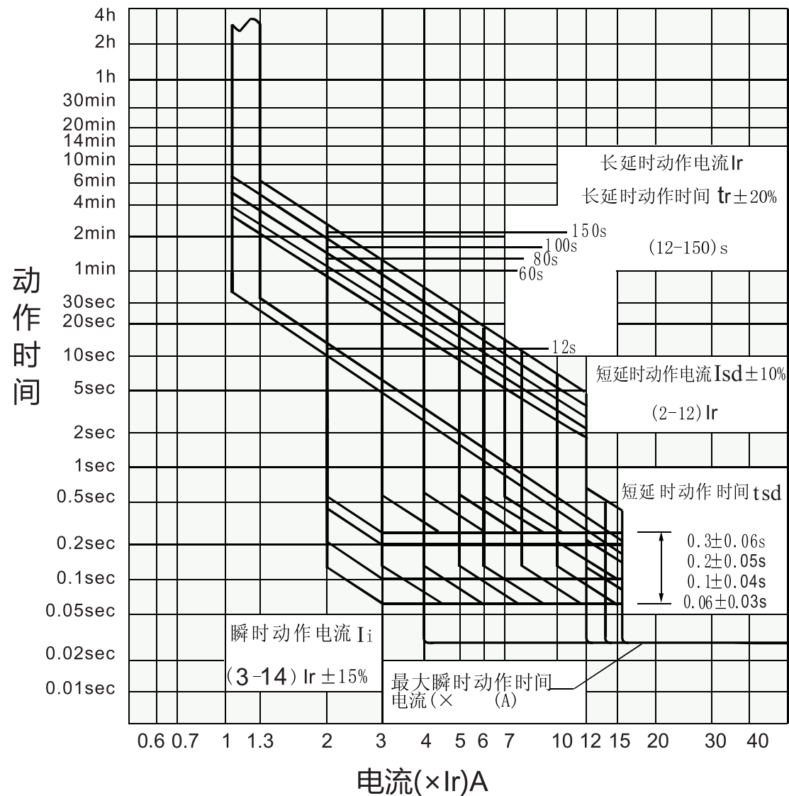
图1 RDM7E-125-800型脱扣特性曲线
