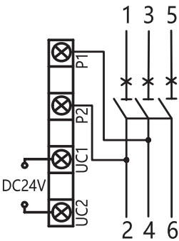
图11 DC24V接线图
