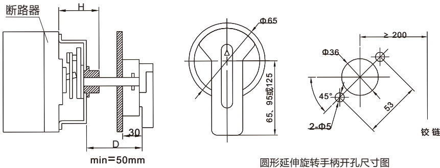
圆形延伸旋转手柄开孔尺寸图
