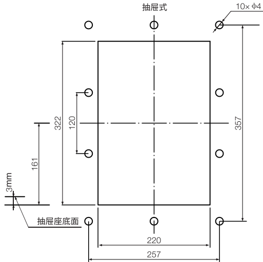
RDW7-1600S抽屉式断路器面板开孔尺寸
