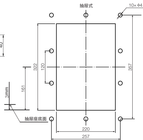
RDW7-1600H抽屉式断路器面板开孔尺寸
