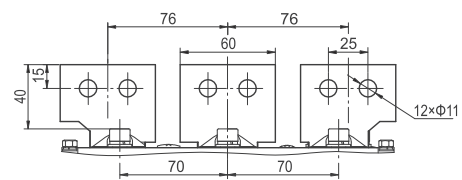
3P水平接线及相间距
