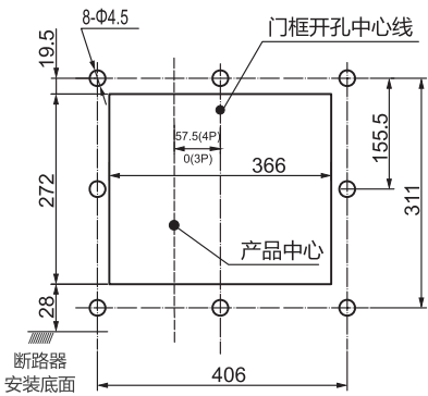
RDW7-4000H固定式断路器面板开孔尺寸
