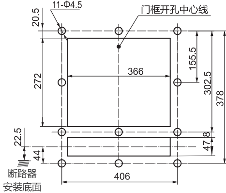
RDW7-6300S抽屉式断路器面板开孔尺寸
