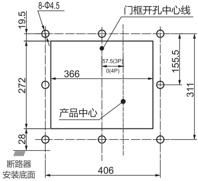
RDW7-6300H固定式断路器面板开孔尺寸
