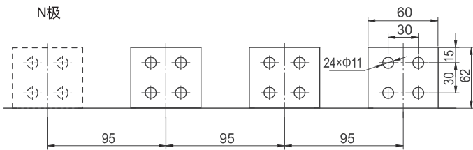
水平接线及相间距
