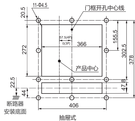
RDW7-4000S抽屉式断路器面板开孔尺寸
