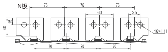
4P水平接线及相间距
