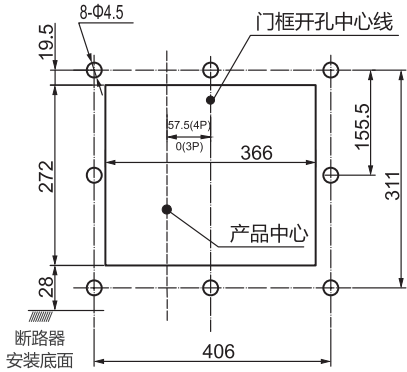
RDW7-4000S固定式断路器面板开孔尺寸
