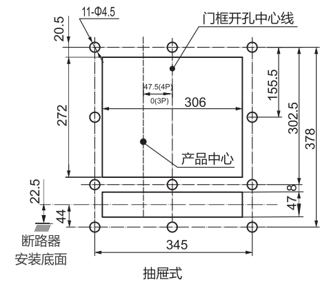
RDW7-2500H抽屉式断路器面板开孔尺寸
