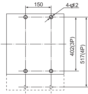
安装尺寸示意图
