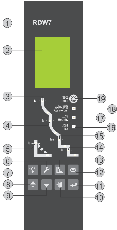
RDW7智能控制器界面
