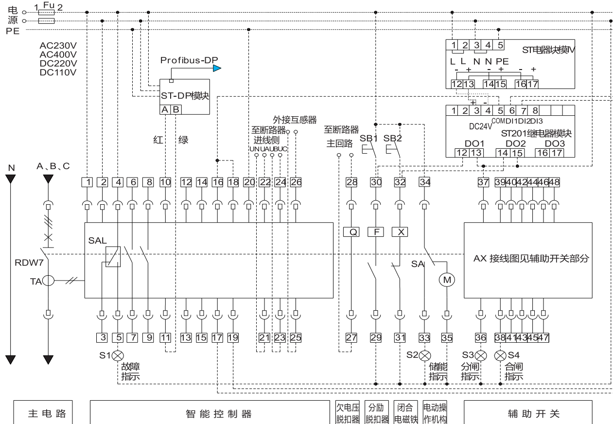
RDW7-1600S,2500~6300S/H H型二次回路接线图
