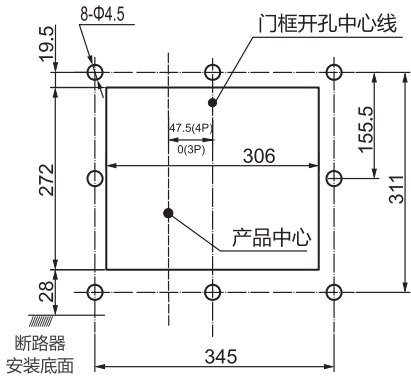
RDW7-2500S固定式断路器面板开孔尺寸
