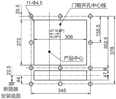
RDW7-2500S抽屉式断路器面板开孔尺寸
