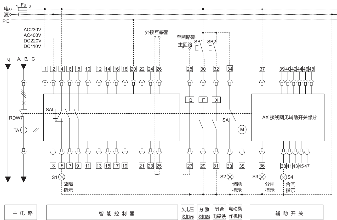
RDW7-1600S,2500~6300S/H M型二次回路接线图
