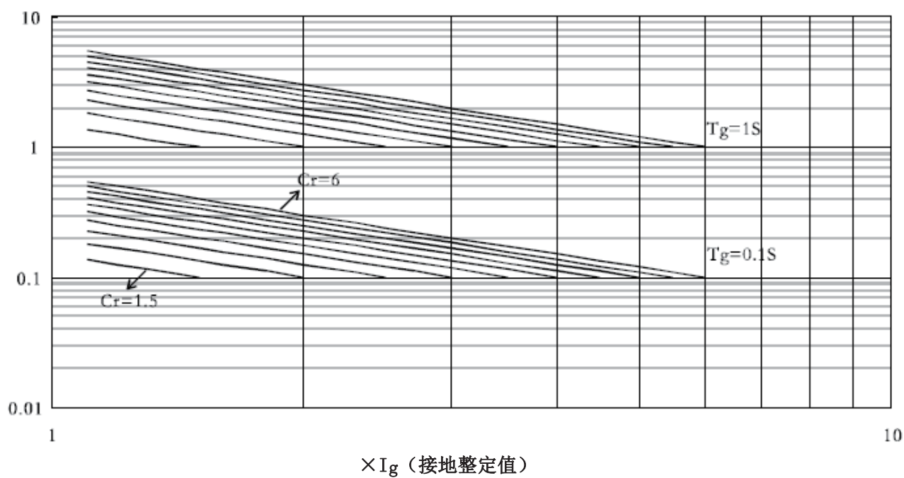
接地保护
