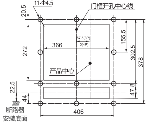
RDW7-6300H抽屉式断路器面板开孔尺寸
