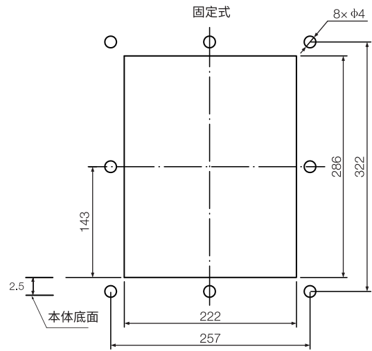
RDW7-1600S固定式断路器面板开孔尺寸
