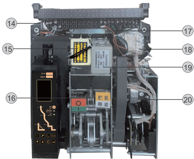
断路器本体
