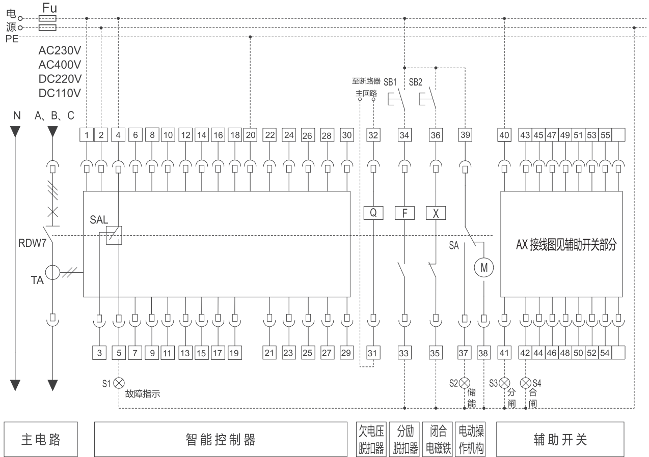
RDW7-1600H M型二次回路接线图
