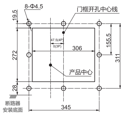
RDW7-2500H固定式断路器面板开孔尺寸
