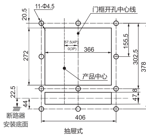
RDW7-4000H抽屉式断路器面板开孔尺寸
