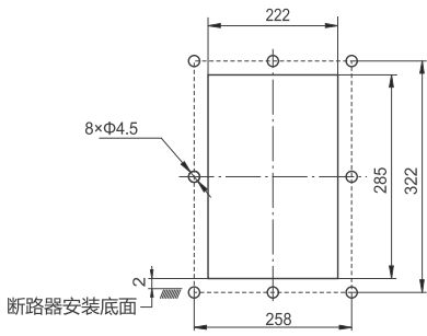
RDW7-1600H固定式断路器面板开孔尺寸
