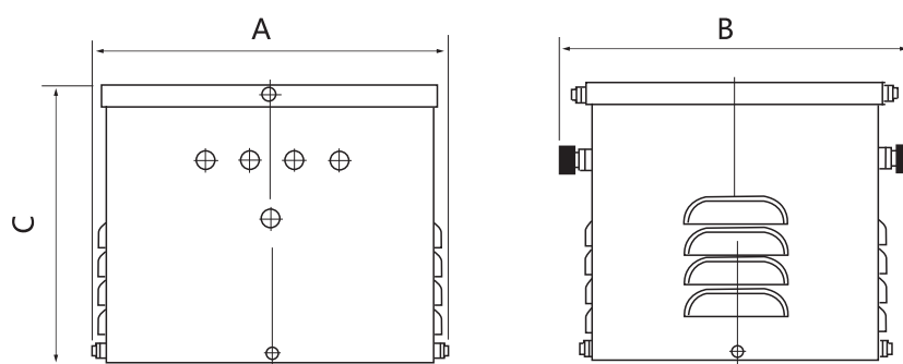
图2 防护式 0.5~20kVA
