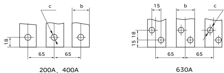
正面操作的安装尺寸和外形尺寸
