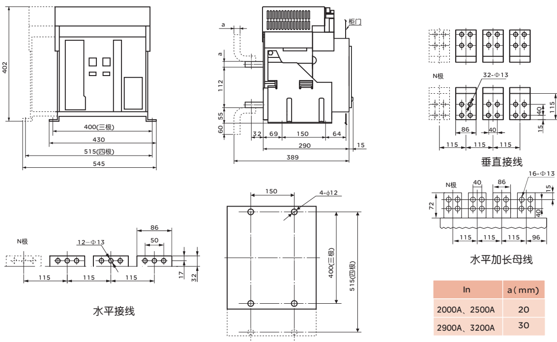
图16 RDW1-3200/3P、4P固定式
