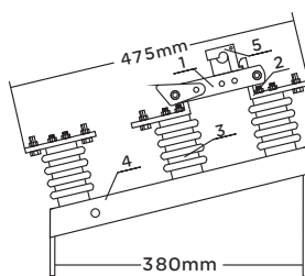
JDW3(GWR1)-0.5G重庆型(图5)
