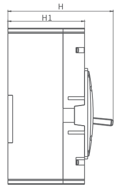
2P外形
