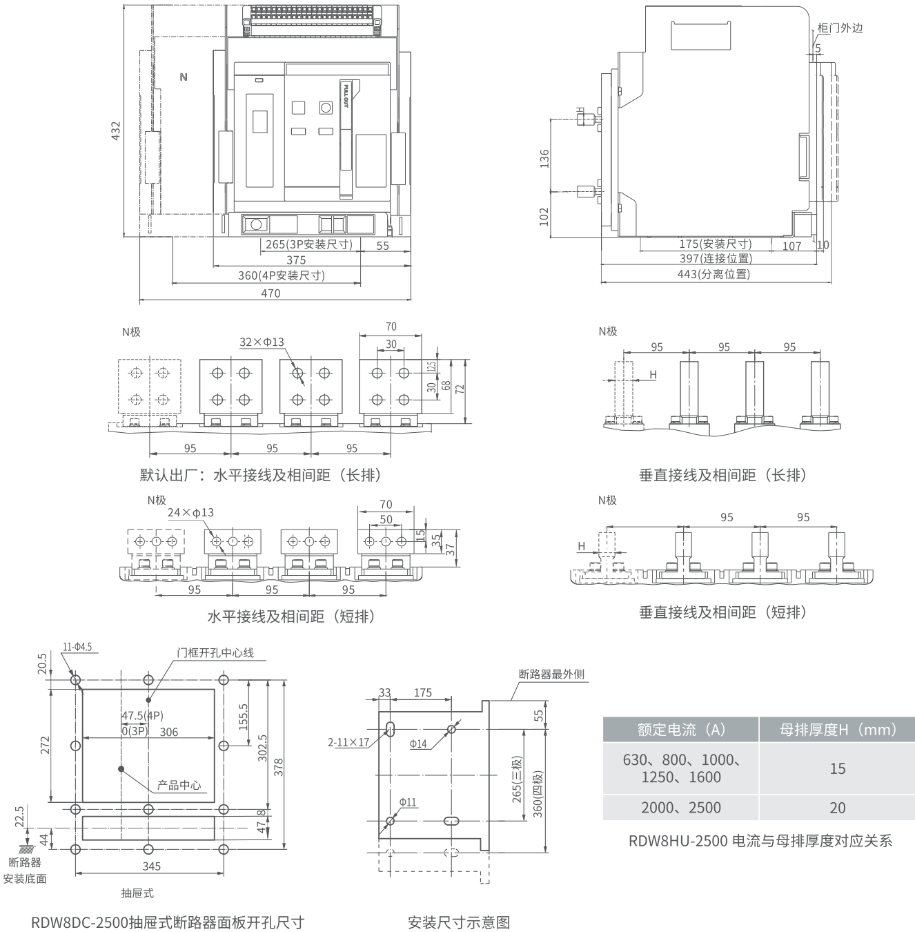
RDW8HU-2500智能型万能式断路器（抽屉式）
