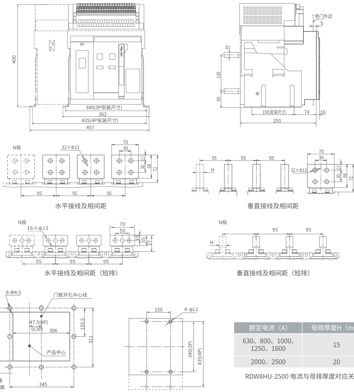
RDW8DC-2500固定式断路器面板开孔尺寸
