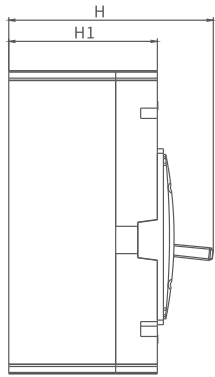
3P外形
