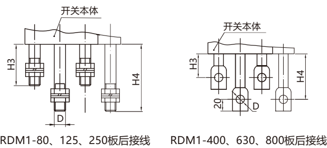
图8 RDM1系列板后接线外形及安装尺寸
