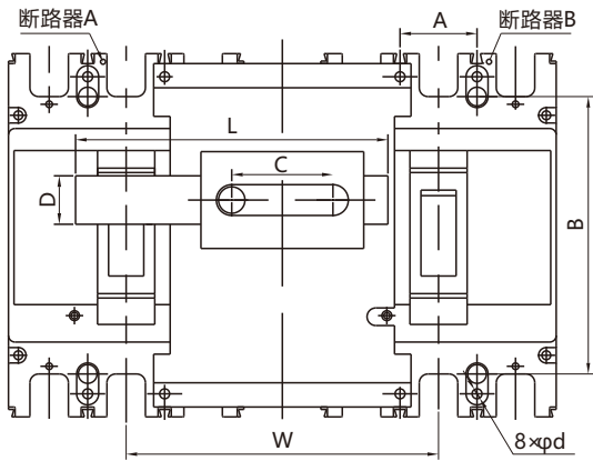
图6 机械连锁机构尺寸图
