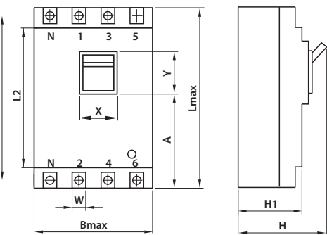
图1 RDL20漏电断路器的外形及安装尺寸
