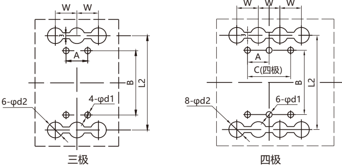
图9 RDM1系列板后接线安装板开孔尺寸
