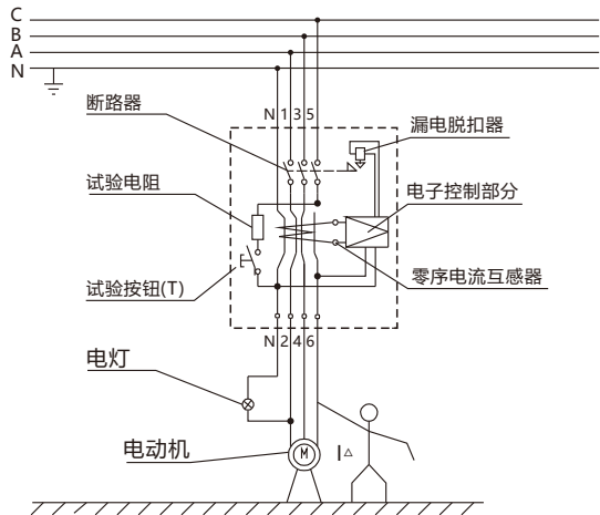
图1 工作原理图
