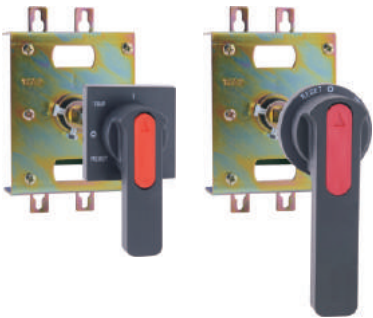
旋转手柄的分类
