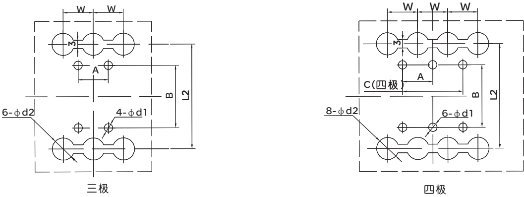
RDM5系列板后接线安装板开孔尺寸
