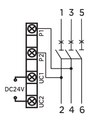
DC24V接线图
