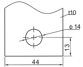
RDM5L-800
