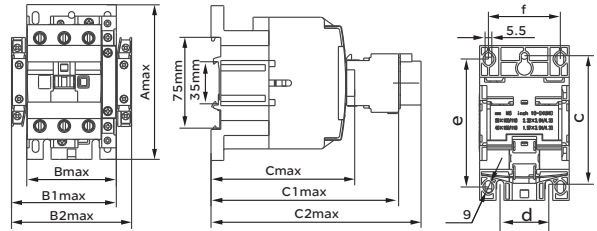
图6 RDC5-40 ~ 95
