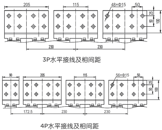
RDW5-6300H接线尺寸
