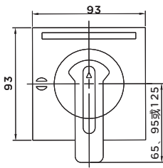
方形延伸旋转手柄开孔尺寸图
